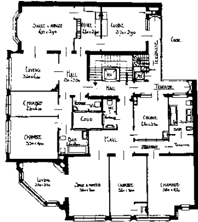
626. Lombardstraat nr. 14-16 (1935). Plattegrond (Le Document, 1939, 5, p. 80).
