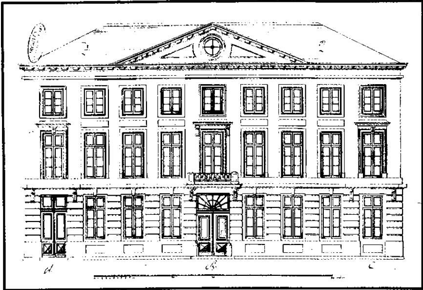
537. Koningsstraat nr. 72. Voormalig «Hotel de Lannoy», later «Hotel de Ligne». Gevelopstand (A.R., Kaarten en plannen in handschrift, 1733).
