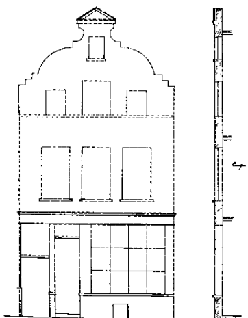
562. Korte Beenhouwersstraat nr. 25-29. Bouwaanvraag (1852), (S.A.B., O.W., 8089).
