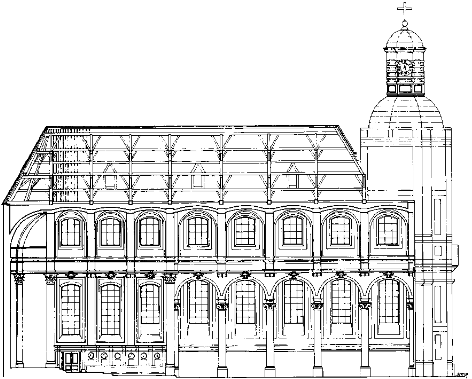
XXIX. Nieuwstraat. Parochiekerk O.-L.-Vrouw van de Finistère. Langsdoorsnede naar architecten M. en P. Mignot (1983).
