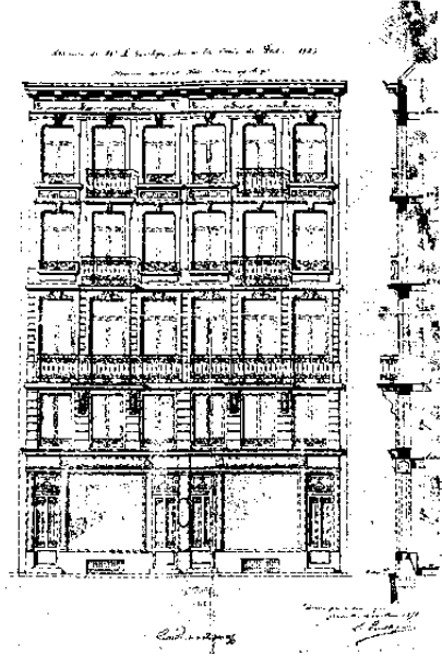
445. IJzerenkruisstraat nr. 15-17, 19-21. Bouwaanvraag (1878), (S.A.B., O.W., 26284).
