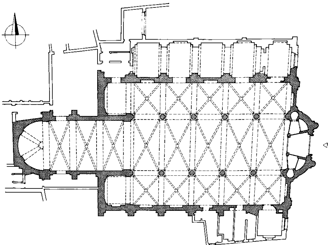
XXX. Nieuwstraat. Parochiekerk O.-L.-Vrouw van de Finistère. Plattegrond naar architecten M. en P. Mignot (1983).
