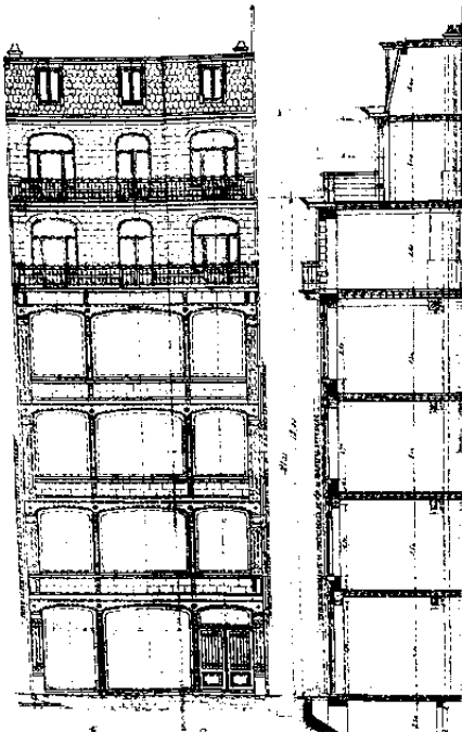
478. Kartuizersstraat nr. 11-11A. Bouwaanvraag (1911). (S.A.B., O.W., 6150).
