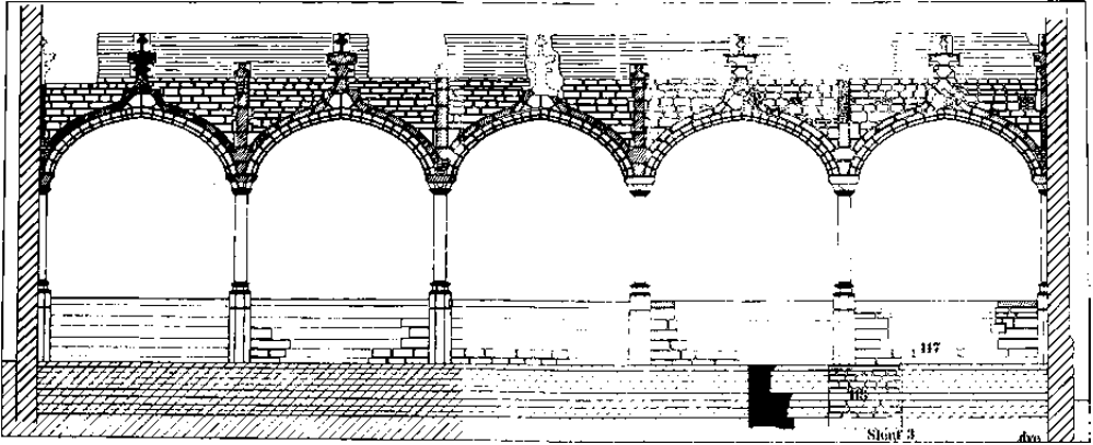
XXI. Koningsplein nr. 11-14. Galerij van het voormalige Hof van Hoogstraten. Opstand door D. Van Eenhooge (1988). Schaal 1 : 160.
