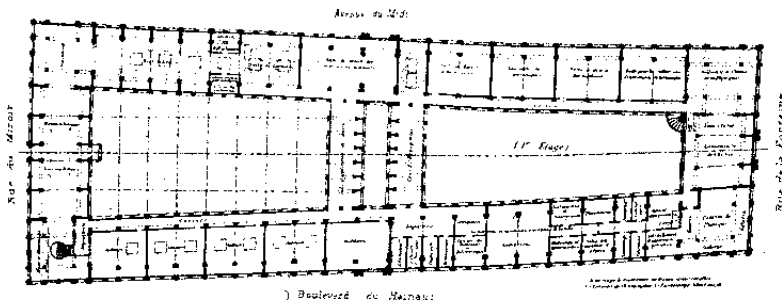
659. Maurice Lemonnierlaan nr. 132-172. Zuidpaleis (1875-1880). Perspectief en plattegrond (S.A.B., P.P., 1032).
