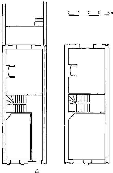
XXIV. Kruitmolenstraat nr. 2 tot 18. Plattegrond naar B. De Meulder (Galerijwoningen te Brussel, dossier 29, eindverhandeling K.U.L., 1982-1983). Schaal 1 : 200.
