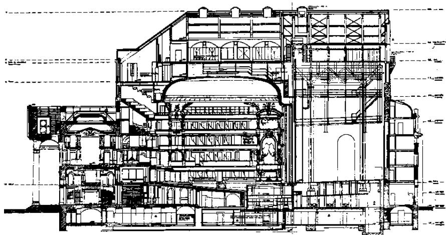
XXVIII. Munt. Koninklijke Muntchouwburg. Langsdoorsnede door architectenbureaus A.2.R.C. en URBAT (1986). Schaal 1 : 600.
