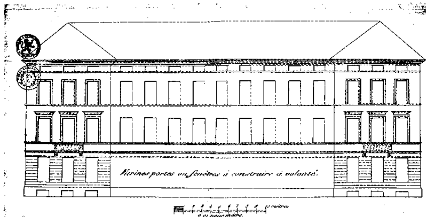
596. Lakensestraat nr. 164 tot 172. Gevelopstand (1835), (S.A.B., O.W., 32189).
