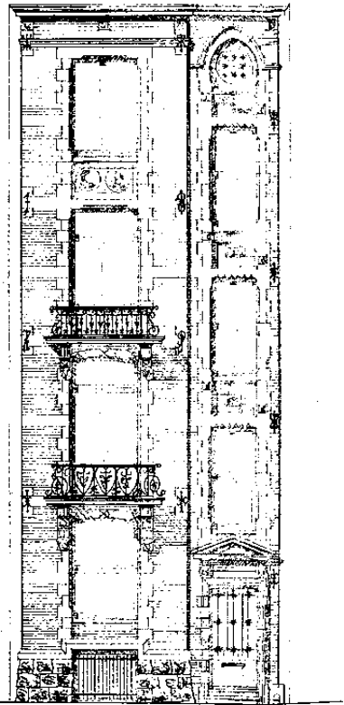
662. Maurice Lemonnierlaan nr. 185. Bouwaanvraag (1879), (S.A.B., O.W., 25187).
