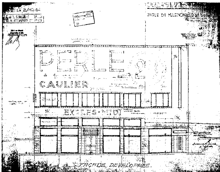
663. Maurice Lemonnierlaan nr. 218. Voormalige brasserie «Express-Midi». Bouwaanvraag (1934), (S.A.B., O.W., 50082).
