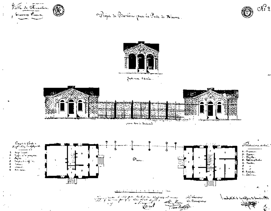
725. Ninoofsepoort. Octrooipaviljoenen. Opstand en plattegrond (1832), (S.A.B., A.A., 1833, vol. 30, resp. 11, pl. 271).
