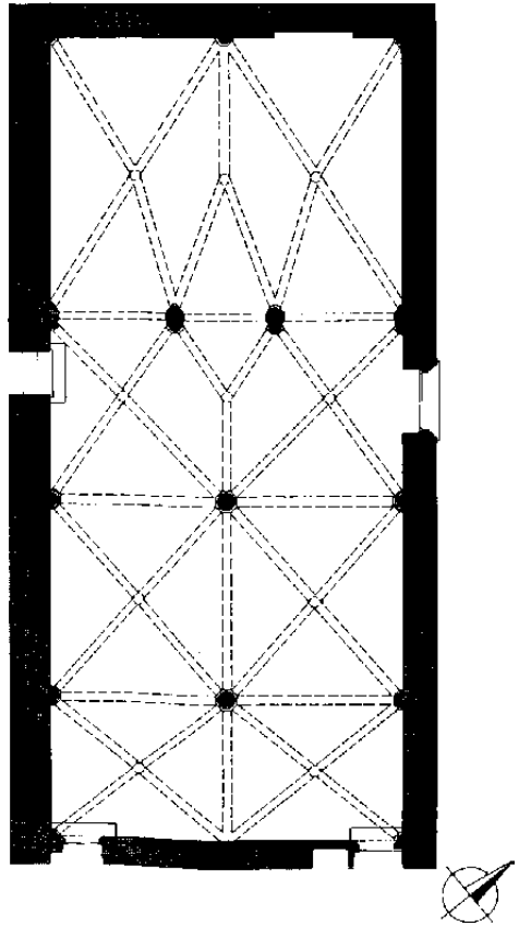
XXV. Kunstberg. St.-Joriskapel. Plattegrond. Schaal 1 : 200.
