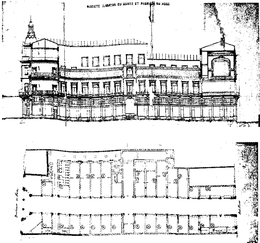
727. Noorddoorgang. Langsdoorsnede en plattegrond (1881), (S.A.B., O.W., 6139).
