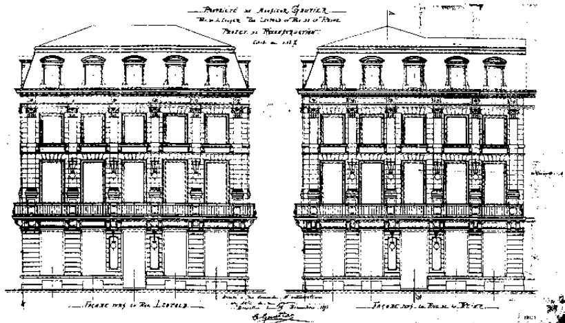
609. Leopoldstraat nr. 2. Bouwaanvraag (1893), (S.A.B., O.W., 10472).
