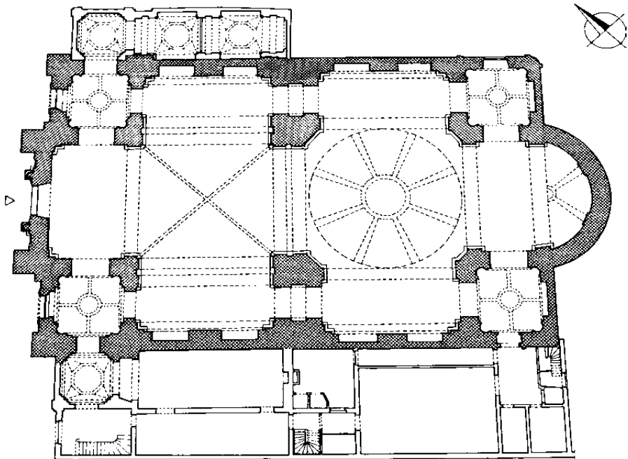
XXVII. Minimenstraat. Parochiekerk St.-Jan en St.-Stefaan ter Minimen. Plattegrond naar architecten E. Cels (1862-1868) en F. Malfait (1923), (S.A.B., N.P.P., C 11).
