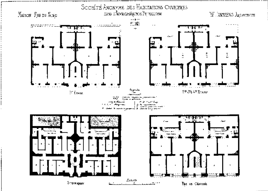
731. Noordstraat nr. 3-11 (1875). Plattegrond (L'Emulation, 1879, pl. 24).
