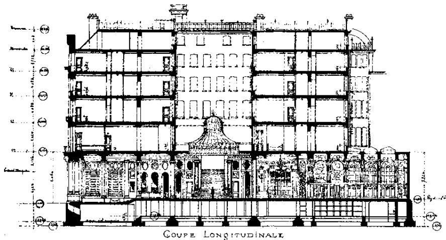
547. Koningsstraat nr. 103. Z.g. «Hotel Astoria». Langsdoorsnede (1909), (S.A.B., O.W., 3899).
