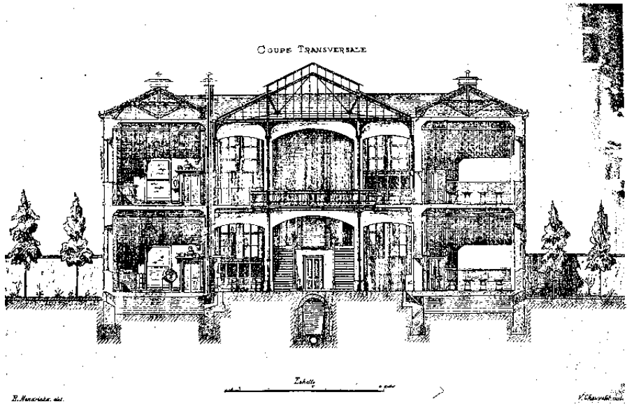
658. Maurice Lemonnierlaan nr. 110. Voormalige «Ecole Modèle» (1873-1875) Dwarsdoorsnede (L'Emulation, 1879, pl. 42).
