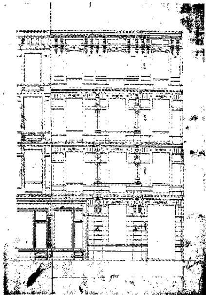
500. Kleerkopersstraat nr. 36. Bouwaanvraag (1865), (S.A.B., O.W., 11690).
