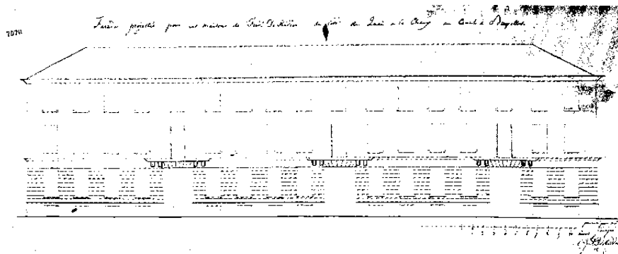
370. Handelskaai nr. 5 tot 11. Bouwaanvraag (1820), (S.A.B., O.W., 7970).
