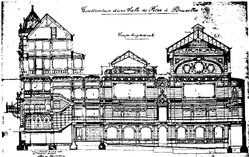
417. Hoogstraat nr. 205-207. Z.g. «Palais Minerva». Langsdoorsnede (1908), (S.A.B., O.W., 5407).
